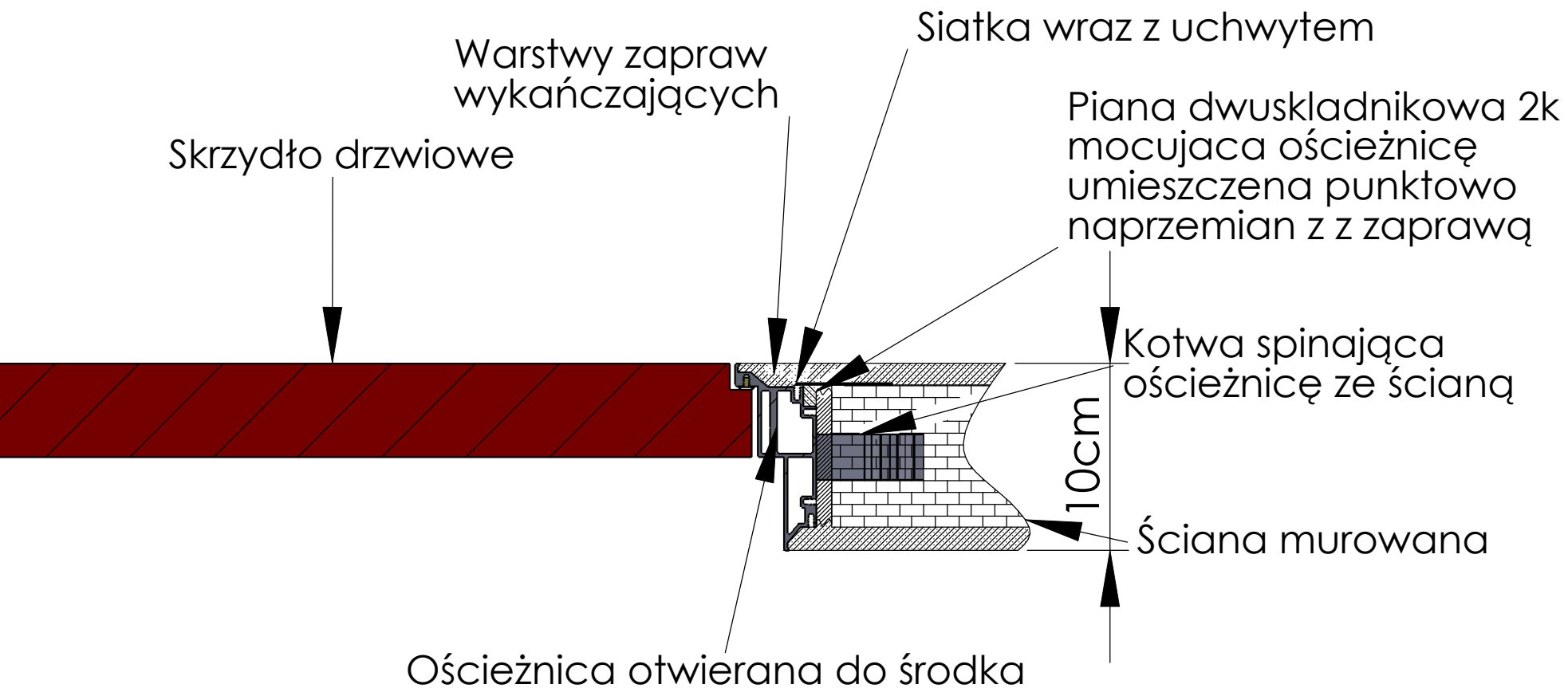
Rys. 01 - Posadowienie ościeżnicy do środka w ścianie murowanej 10cm
