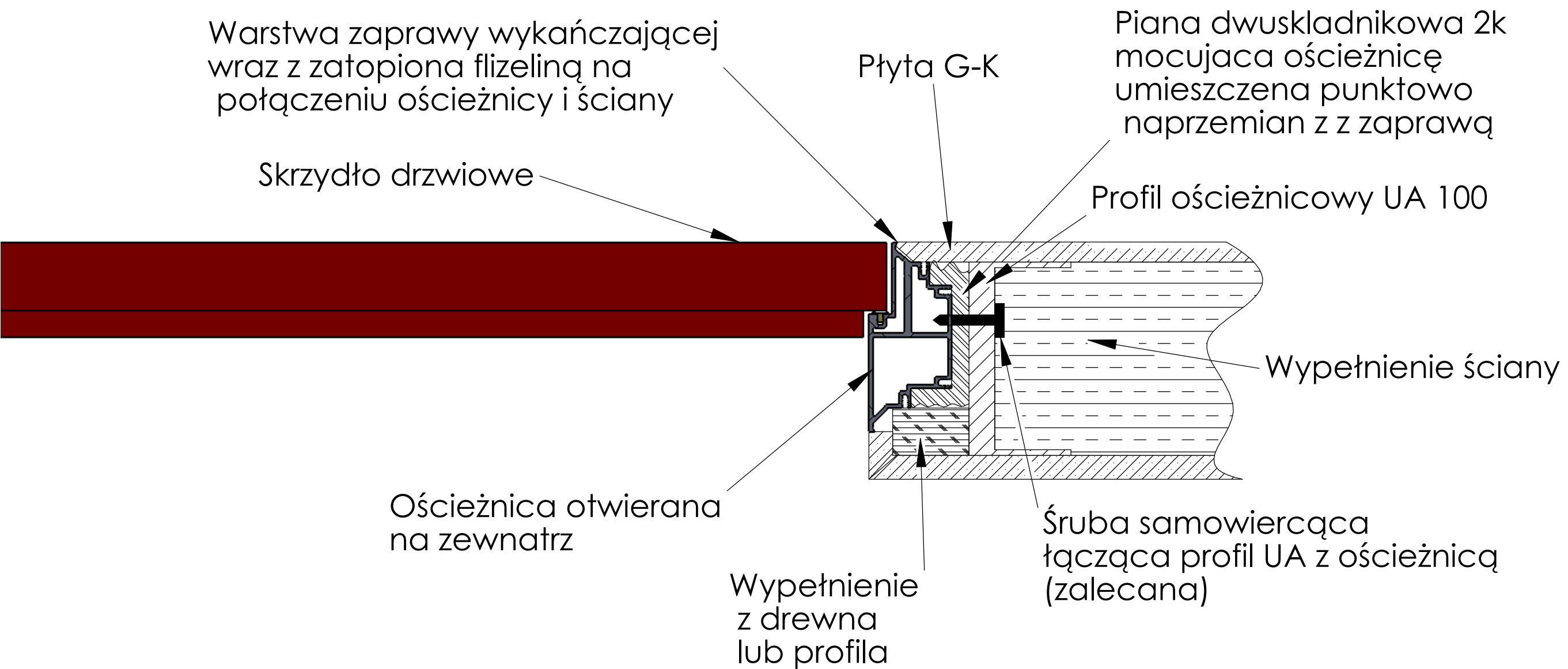
Rys. 08- Posadowienie ościeżnicy na zewnątrz w ścianie 1x GK na profilu UA 100, ściana ponad 10cm
