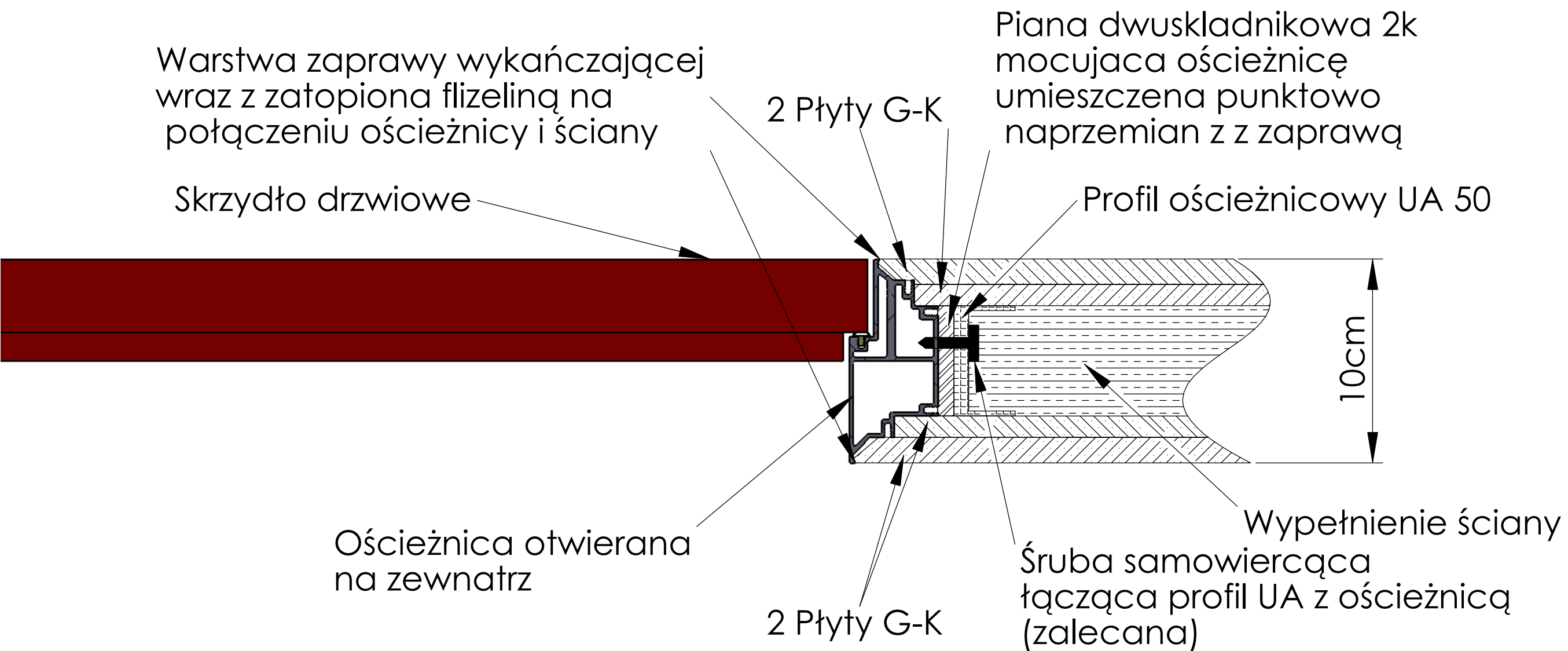
Rys. 11- Posadowienie ościeżnicy na zewnątrz w ścianie 2x GK na profilu UA 50 , ściana 10cm
