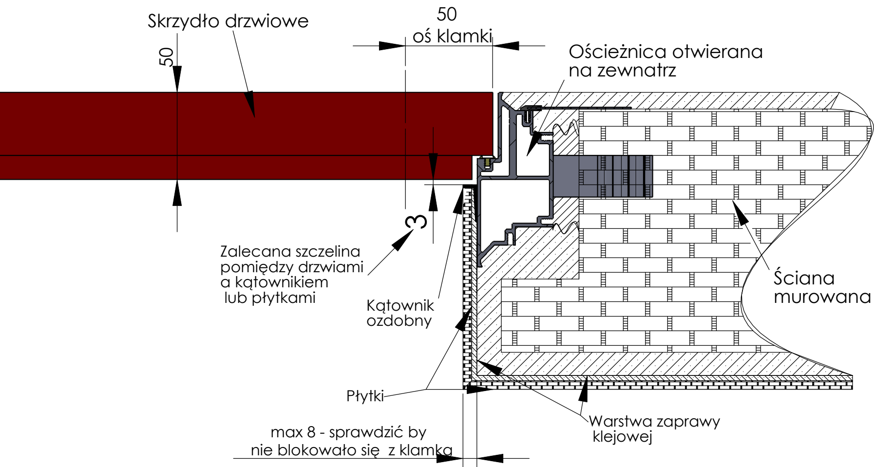
Rys. 14- Wykończenie ościeżnicy otwieranej na zewnątrz płytka
