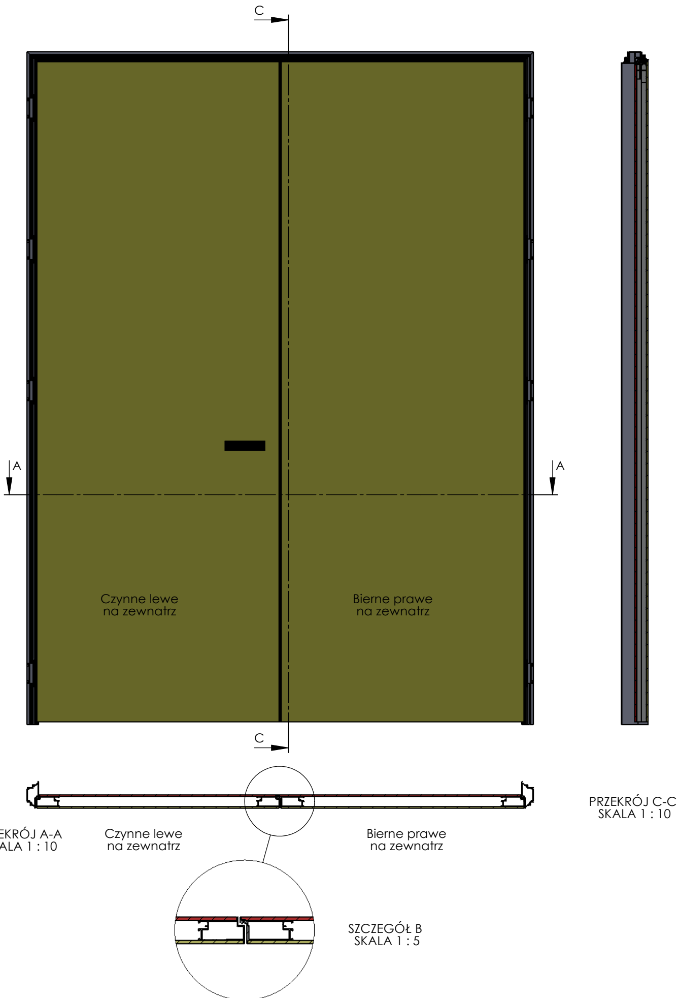
Rys. 23. Drzwi podwójne czynne lewe na zewnątrz, bierne prawe na zewnątrz
