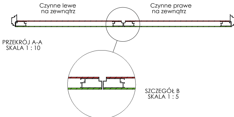
Rys. 25. Drzwi szafowe, czynne, lewe na zewnątrz czynne, prawe na zewnątrz
