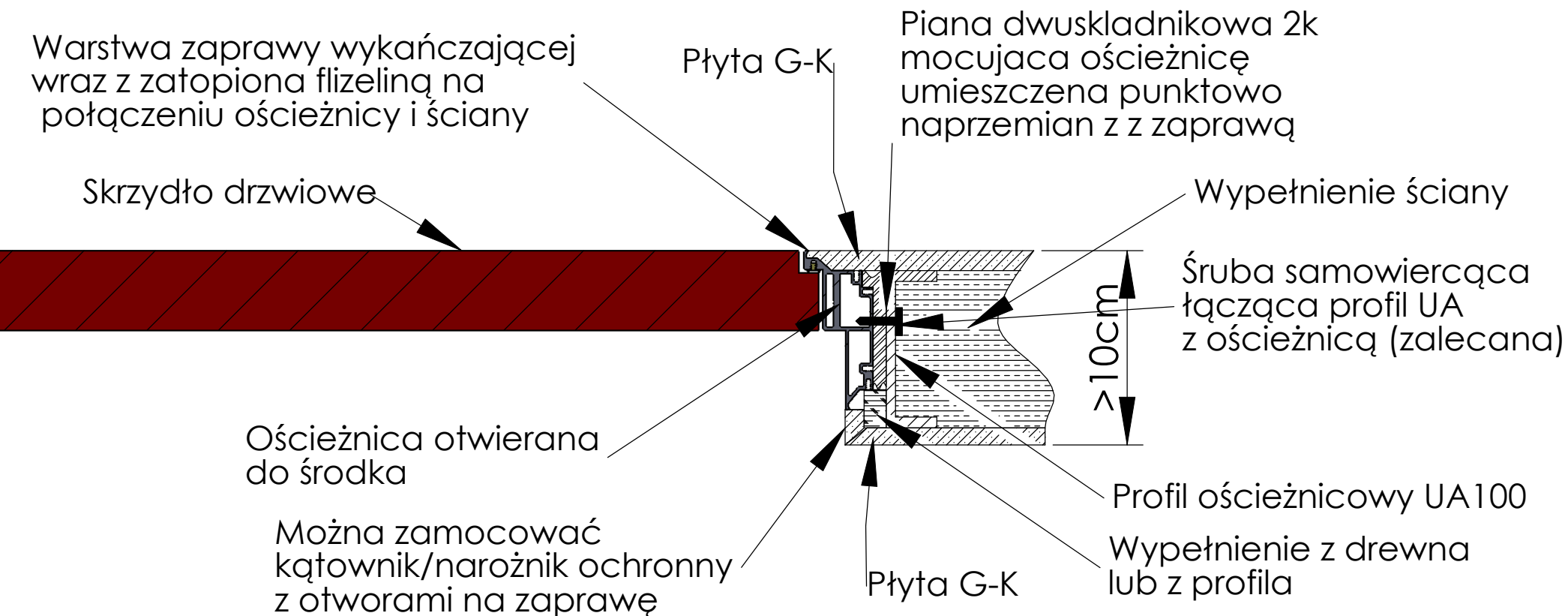
Rys. 06- Posadowienie ościeżnicy do środka w ścianie 1xGK na profilu UA 100 ściana ponad 10cm
