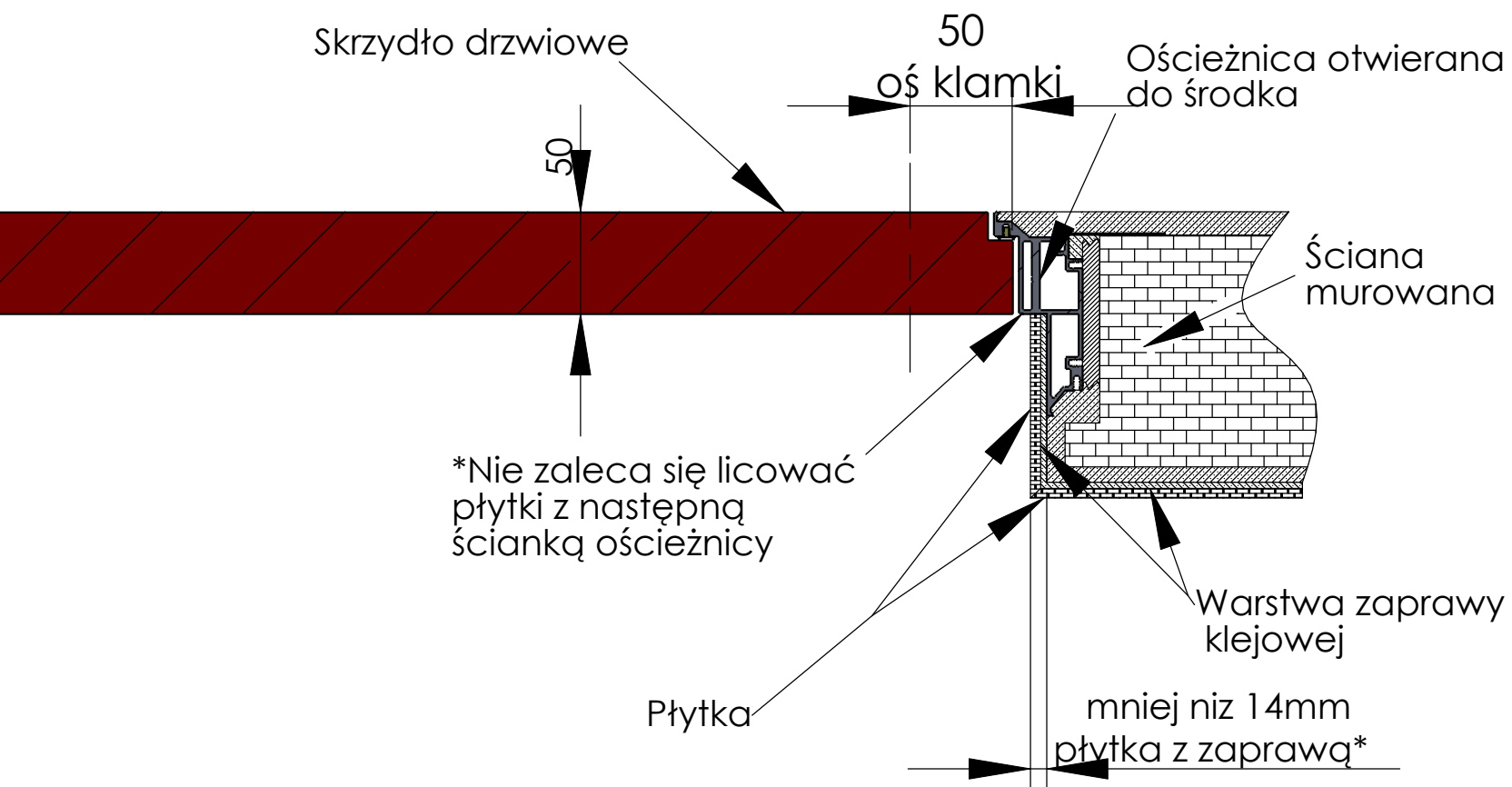
Rys. 13-Wykończenie ościeżnicy otwieranej do środka płytką
