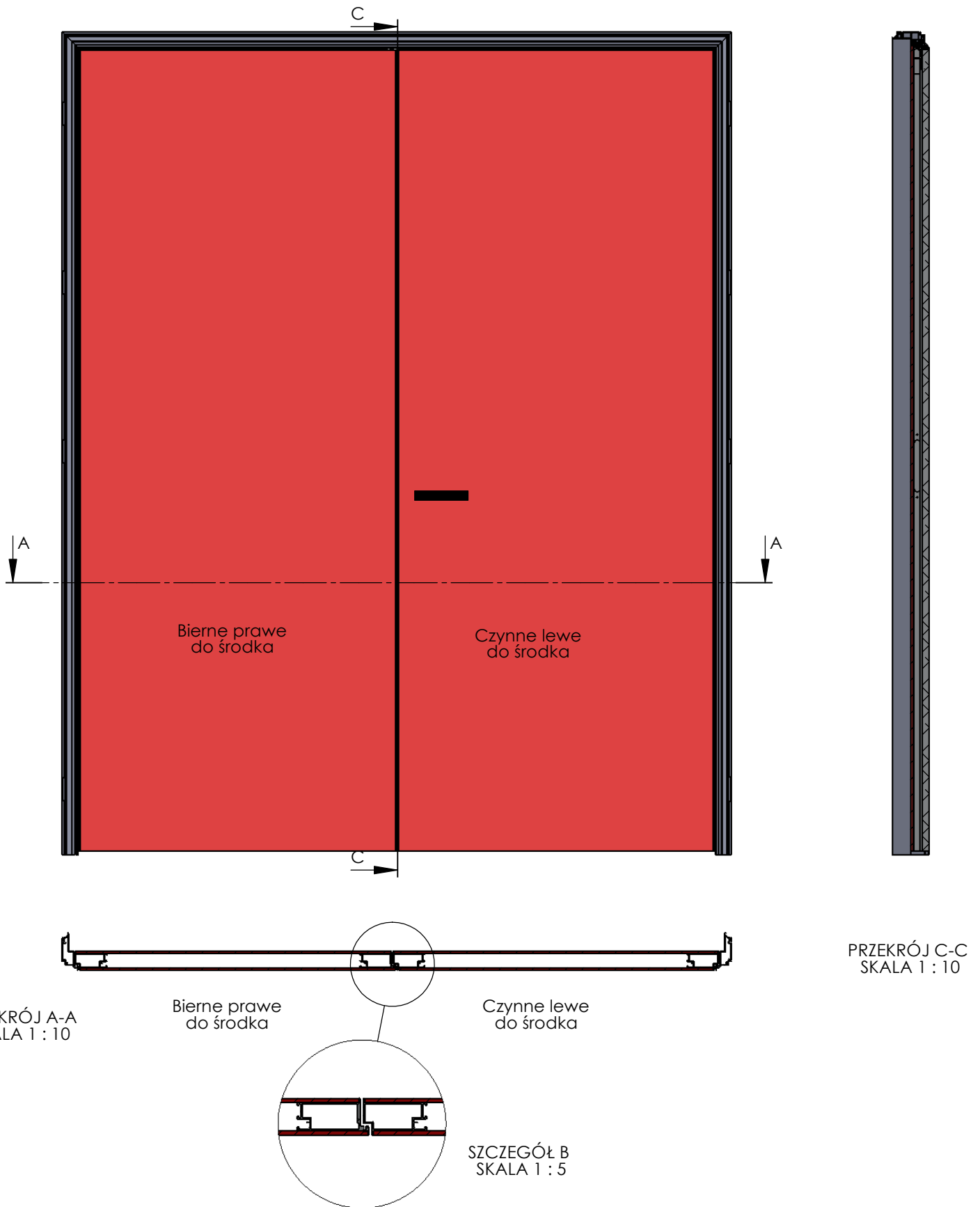
Rys. 21. Drzwi podwójne czynne lewe środek, bierne prawe środek
