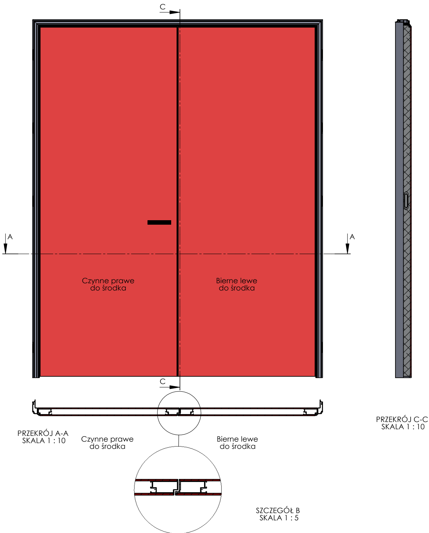
Rys. 22. Drzwi podwójne bierne lewe środek, czynne prawe środek
