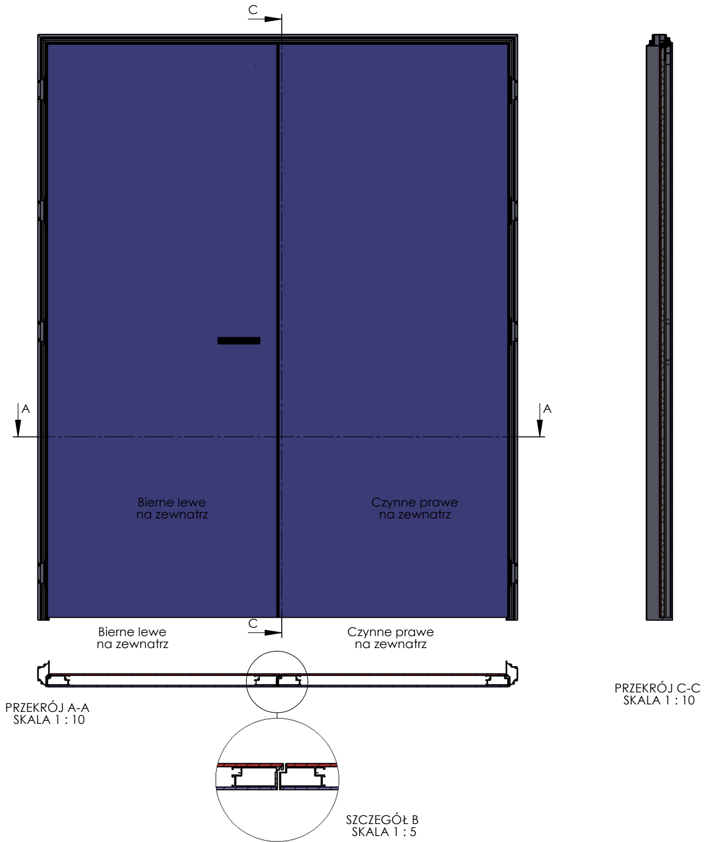
Rys. 24. Drzwi podwójne bierne lewe na zewnątrz, czynne prawe na zewnątrz
