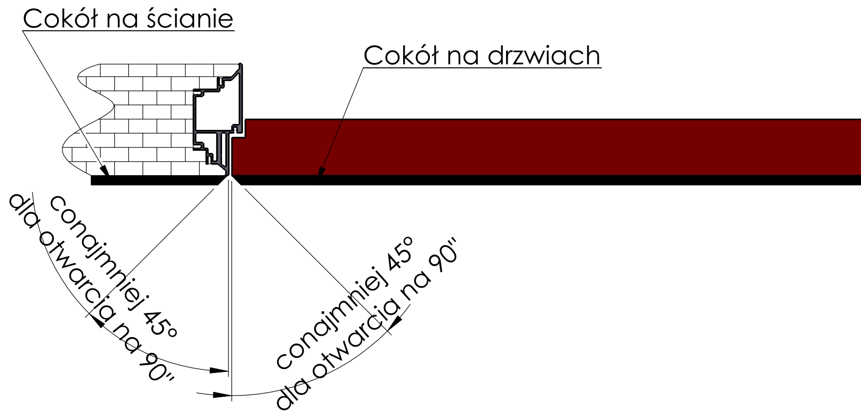
Rys. 25 Cokół na skrzydle i ościeznicy otwieranej na zewnątrz
