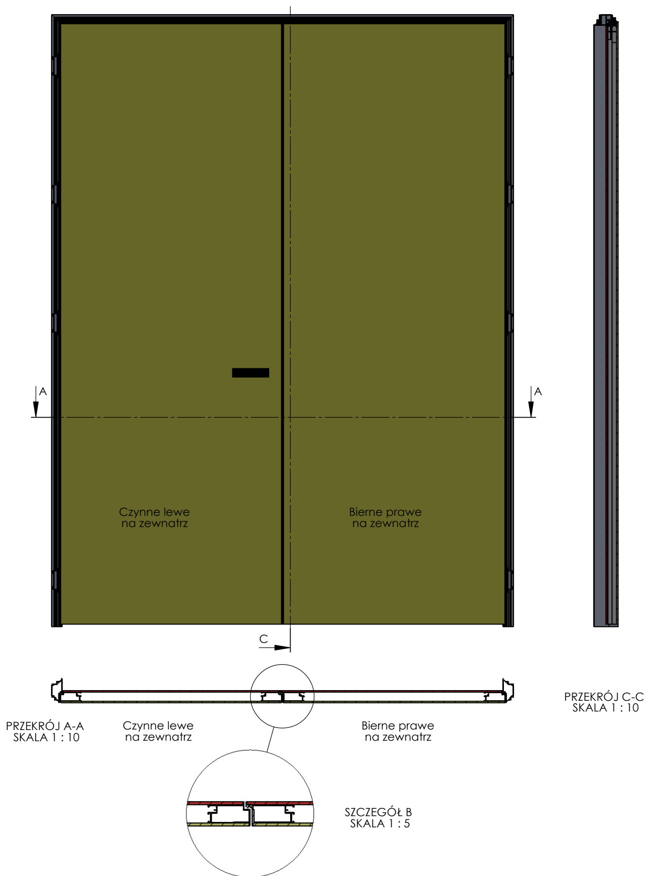
Rys. 2 – SCHEMAT DRZWI PIU PODWÓJNYCH NA ZEWNĄTRZ – LEWE CZYNNE, PRAWY BIERNE
