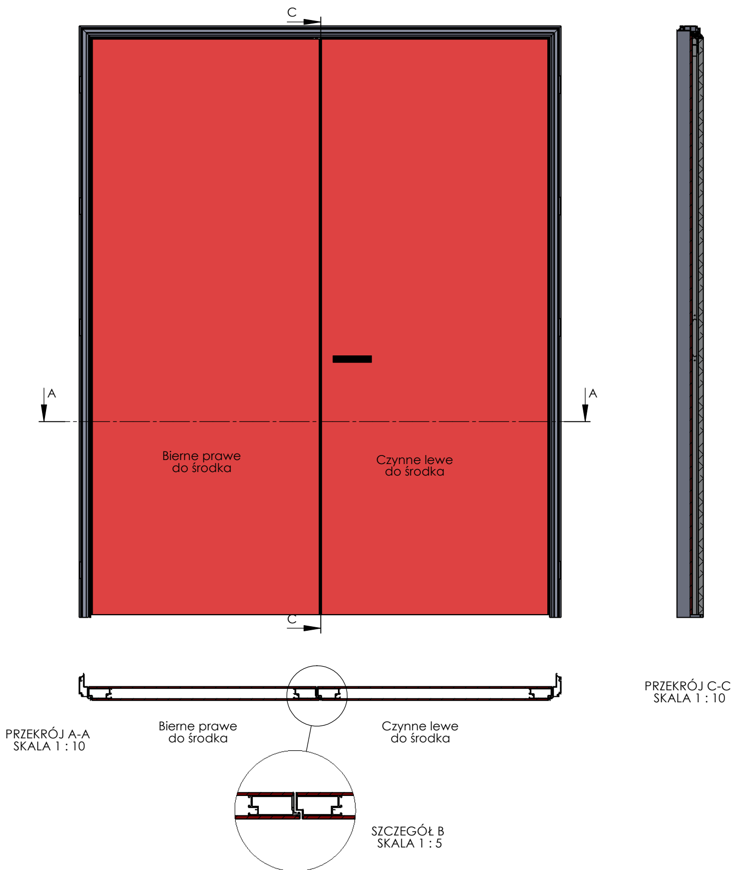
Rys. 1 – SCHEMAT DRZWI PIU PODWÓJNYCH DO ŚRODKA – LEWE CZYNNE, PRAWY BIERNE
