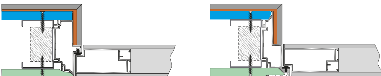
Rys. 8 – OBRÓBKĄ OŚCIEŻNICY PŁYTKĄ CERAMICZNĄ
